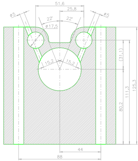
Schnitt A-A (90° gedreht gezeichnet)
